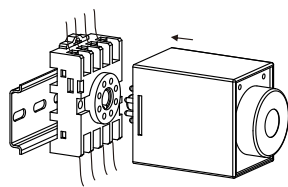
(9) 导轨式安装：装上继电器， 上插的凸台应对准底座的凹槽
