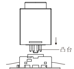
(3) 装置式安装: 装上继电器, 上插的凸台应对准底座的凹槽
