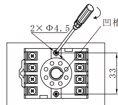
(1) 装置式安装: 拧紧安装螺钉
