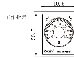
HHS8-1(AH3-1)、HHS8(AH3-2)、 HHS8C(AH3-3)、HHS8G(AH3-2)释放延时
